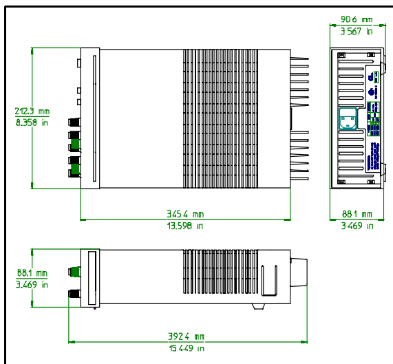
Figure 1. Schéma d'encombrement
