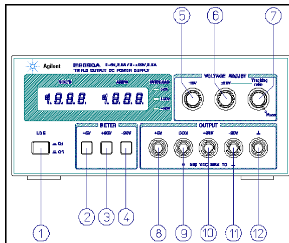
Abbildung 2. Bedienelemente und Anzeigen auf der Frontplatte
