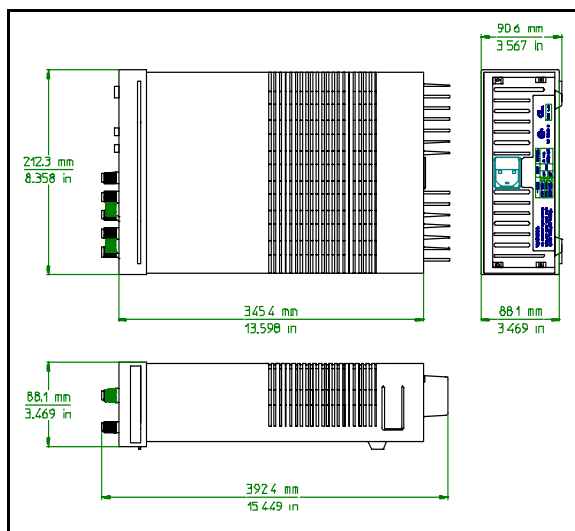
圖 1 概要圖表
