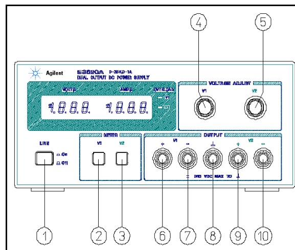
Figure 2. Contrôles et voyants de la face avant
