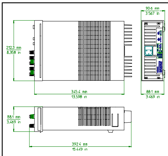
Abbildung 1. Maßskizze
