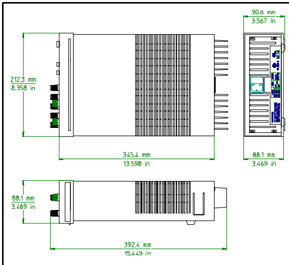
그림 1. 외형도
